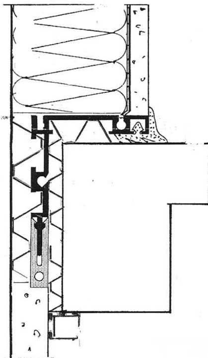
LANCO-ZARGE Profil 40-W für Leibungsdämmung bis ca. 50 mm
