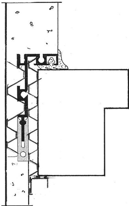
LANCO-ZARGE Profil 20-W für Putz ohne Dämmung
